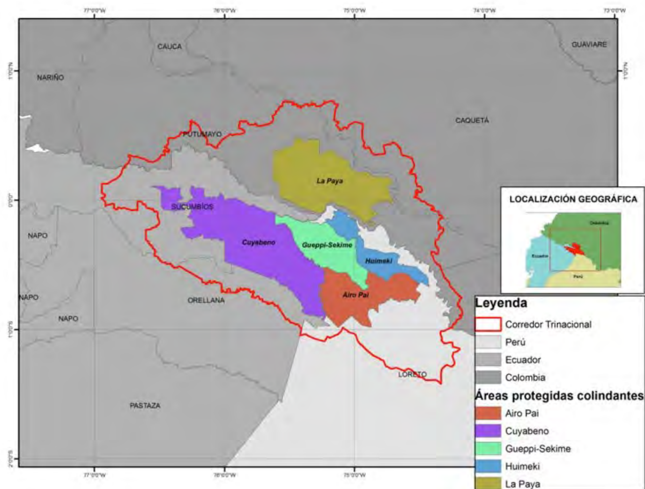
Figura 1: áreas protegidas del Corredor Trinacional, después de la categorización de la zona reservada de Güeppi.
