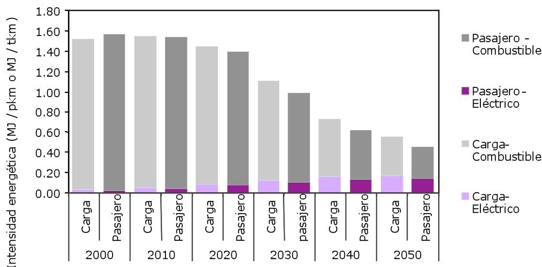
Gráfica 3 - 16 Evolución de la intensidad energética en el sector Transporte.
