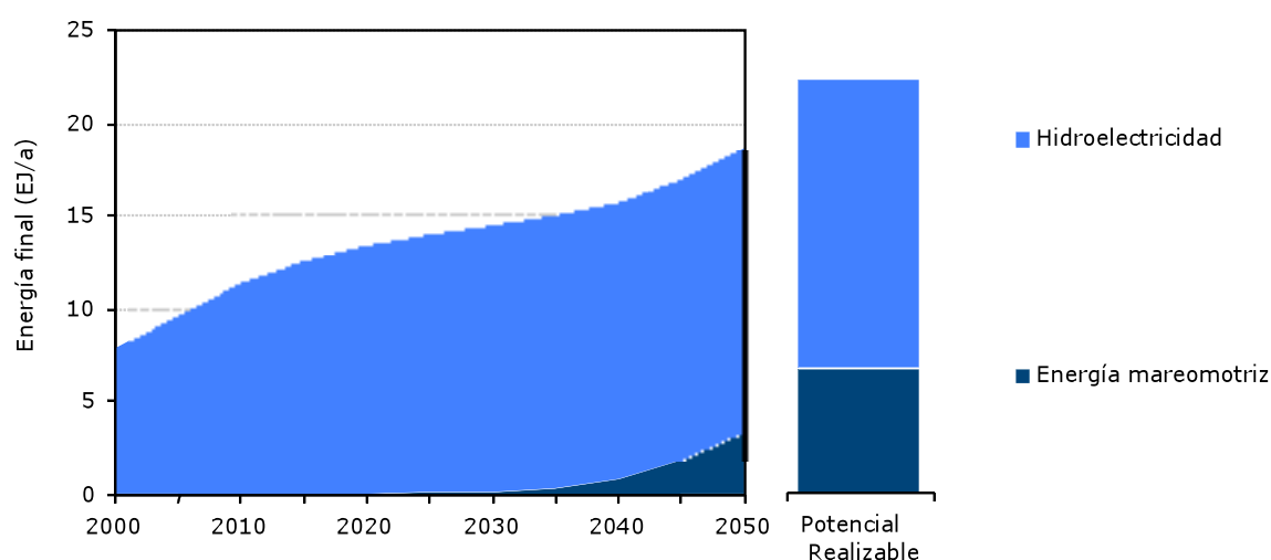
Gráfica 4 – 4 Potencial global de despliegue de energía hidroeléctrica y mareomotriz. (A la izquierda: Evolución del potencial de despliegue en el tiempo; a la derecha: Potencial máximo factible).
