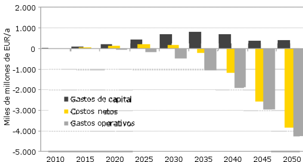
Gráfica 6 - 14 Resultados para el transporte - infraestructura.
