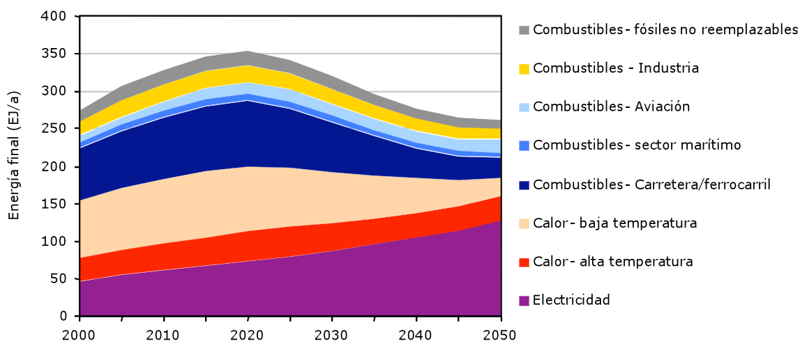
Gráfica 4 – 1 Demanda global de energía en todos los sectores, por tipo de portador de energía.
