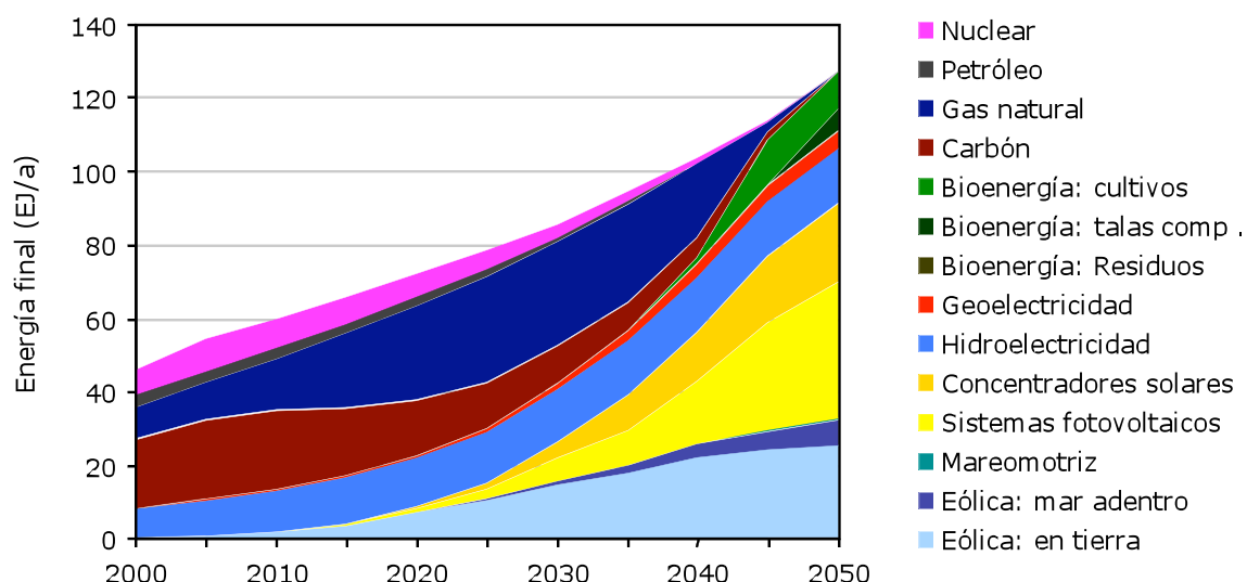
Gráfica 4 – 7 Oferta global de electricidad en el Escenario Energético.
