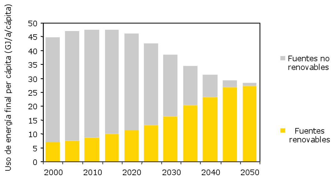
Gráfica 8 - 2 Evolución per cápita de la demanda de energía de fuentes renovables y no renovables.
