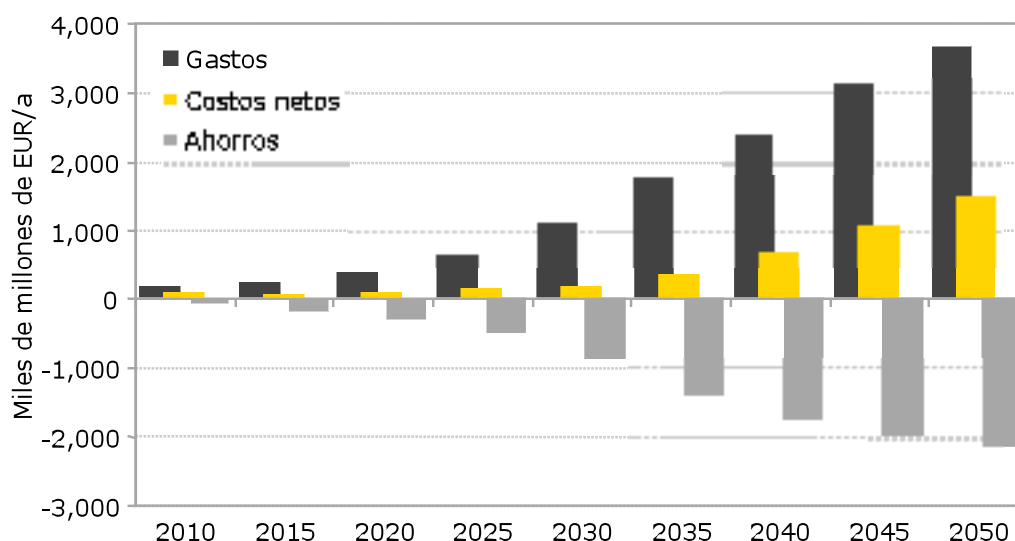
Gráfica 6 - 21 Resultados para calor y combustibles renovables.
