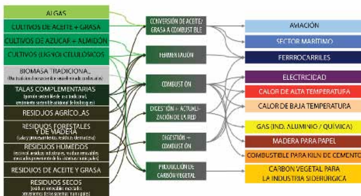
Gráfica 2 – 6 Enfoque sobre bioenergía, mostrando los diferentes tipos de insumos de biomasa y rutas de conversión que resultan en diversos tipos de portadores de energía para cubrir la demanda. 8,9
