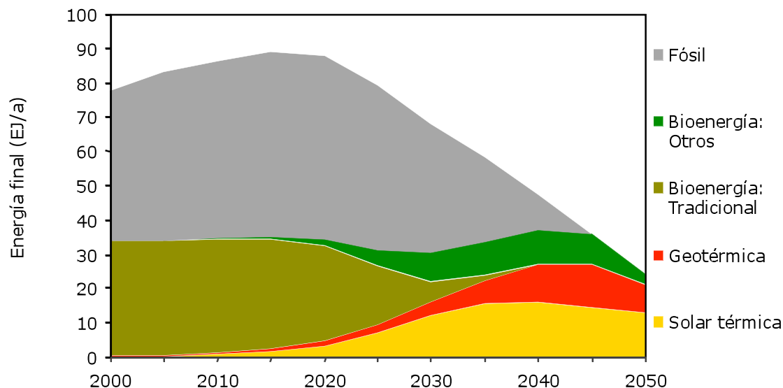
Gráfica 4 – 12 División de opciones de oferta de energía en el sector global de Edificios (sin contar la electricidad).
