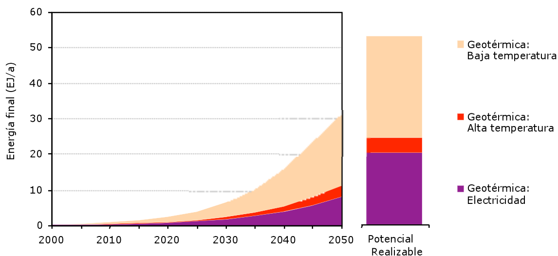
Gráfica 4 – 6 Potencial global de despliegue de la energía geotérmica. (A la izquierda: Evolución del potencial de despliegue en el tiempo; a la derecha: Potencial máximo factible)
