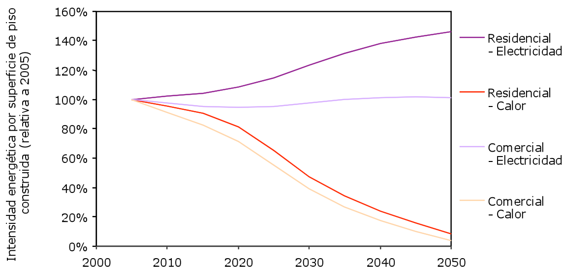
Gráfica 3 – 11 Evolución de la intensidad energética en el sector de Edificios. 16
