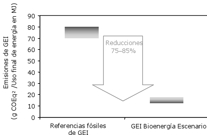
Gráfica 5 – 21 Emisiones de GEI en el Escenario Energético contra referencias de combustibles fósiles para 2050. 60
