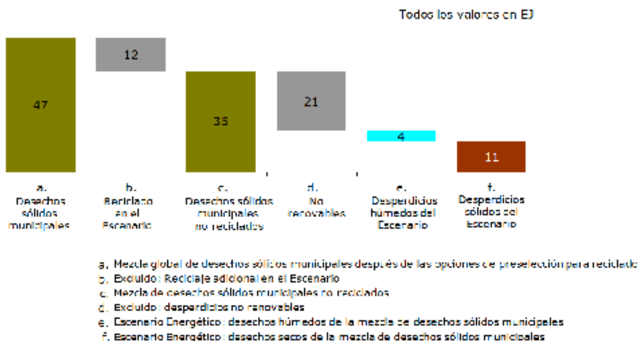
Gráfica 5 – 16 Análisis adicional para el potencial de los desechos sólidos municipales.
