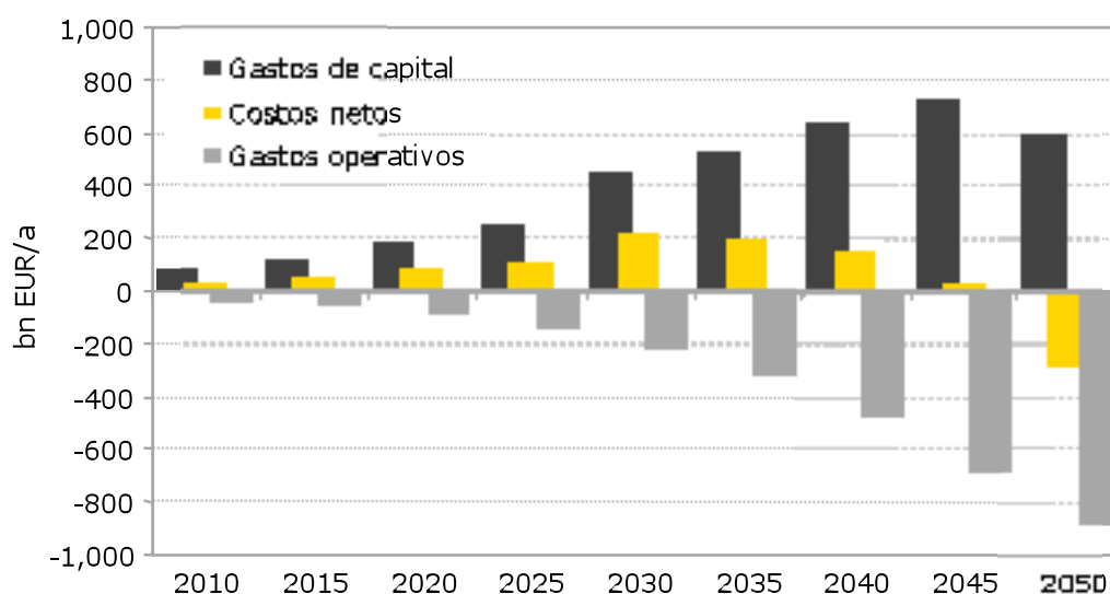
Gráfica 6 - 17 Resultados para electricidad.
