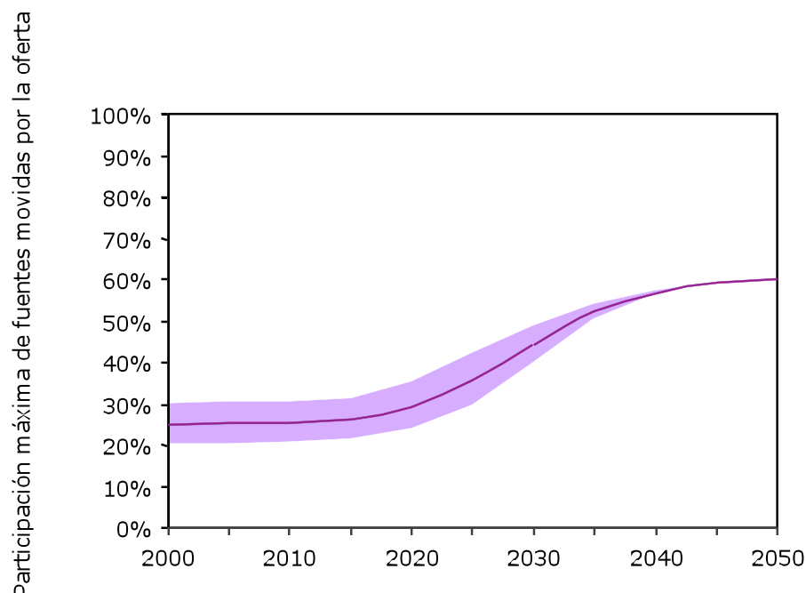
Gráfica 4 – 8 Restricciones impuestas a la energía fotovoltaica y la energía eólica debido a los límites de potencia de las redes eléctricas. El rango representa las diferencias en todas las regiones.
