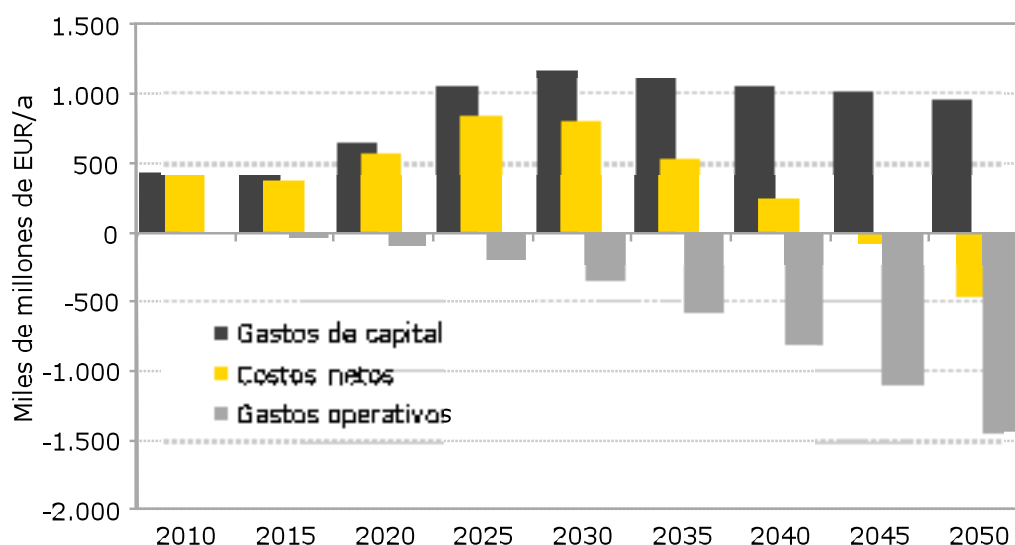
Gráfica 6 - 10 Resultados para edificios.
