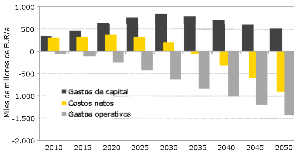
Gráfica 6 - 15 Resultados para el transporte - tecnología vehicular
