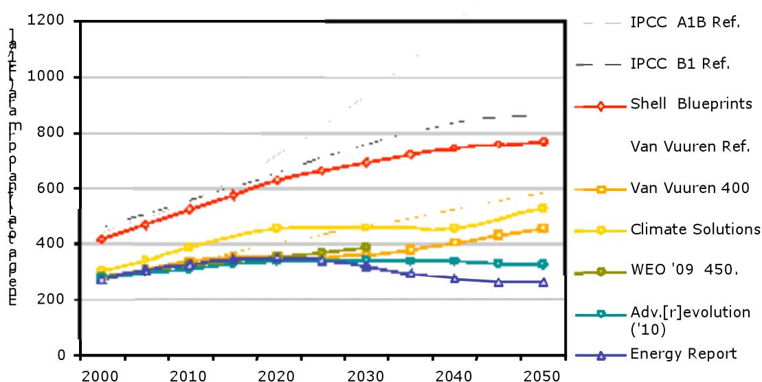
Gráfica 3 – 2 Comparación de la evolución de la demanda global de energía en el Escenario Energético con otros escenarios. Las tres líneas en la parte superior corresponden a energía primaria, las siguientes seis refieren energía final.
