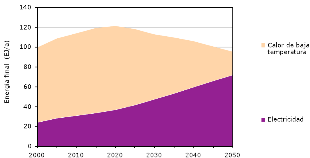
Gráfica 3 - 12 Uso global general de energía en el sector Edificios, por tipo de portador de energía.
