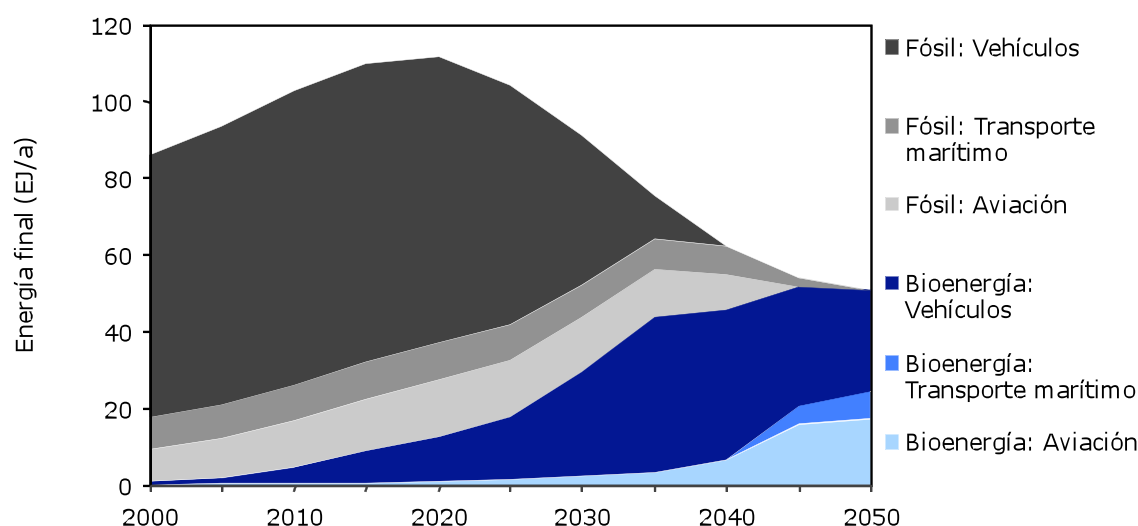
Gráfica 4 – 13 División de las opciones de oferta de energía en el sector global del Transporte (sin contar a la electricidad).
