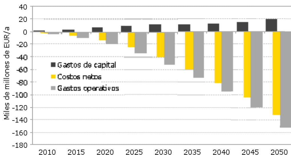
Gráfica 6 – 7 Resultados de la industria (todos los sectores).
