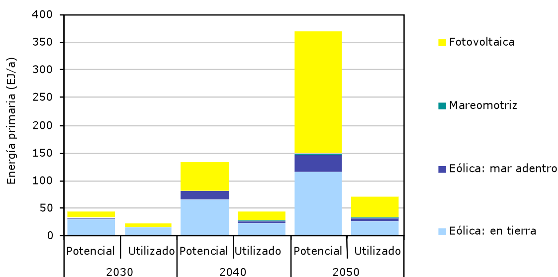
Gráfica 4 – 9 Potencial de despliegue total vs uso real de fuentes de electricidad movidas por la oferta.
