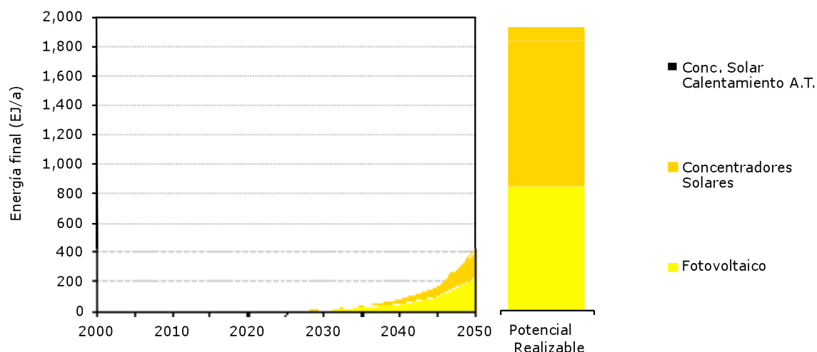
Gráfica 4 – 5 Potencial global de despliegue de sistemas solares para generación de electricidad y calor (con excepción de los sistemas térmicos para edificios). (A la izquierda: Evolución del potencial de despliegue en el tiempo; a la derecha: Potencial máximo factible)
