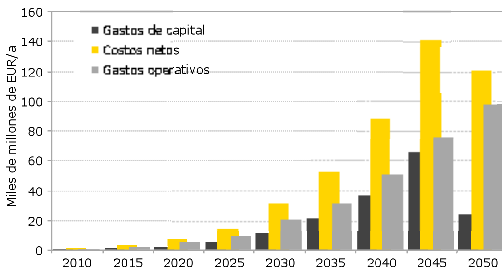
Gráfica 6 - 19 Resultados para redes eléctricas.
