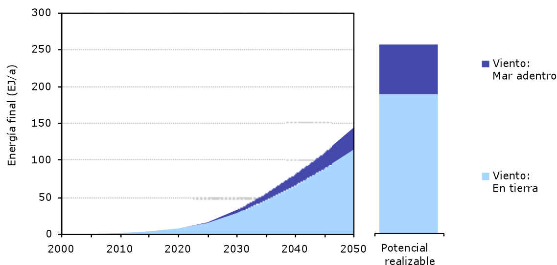
Gráfica 4 – 3 Potencial de despliegue global de energía eólica. (A la izquierda: Evolución del potencial de despliegue en el tiempo; a la derecha: Potencial máximo factible)
