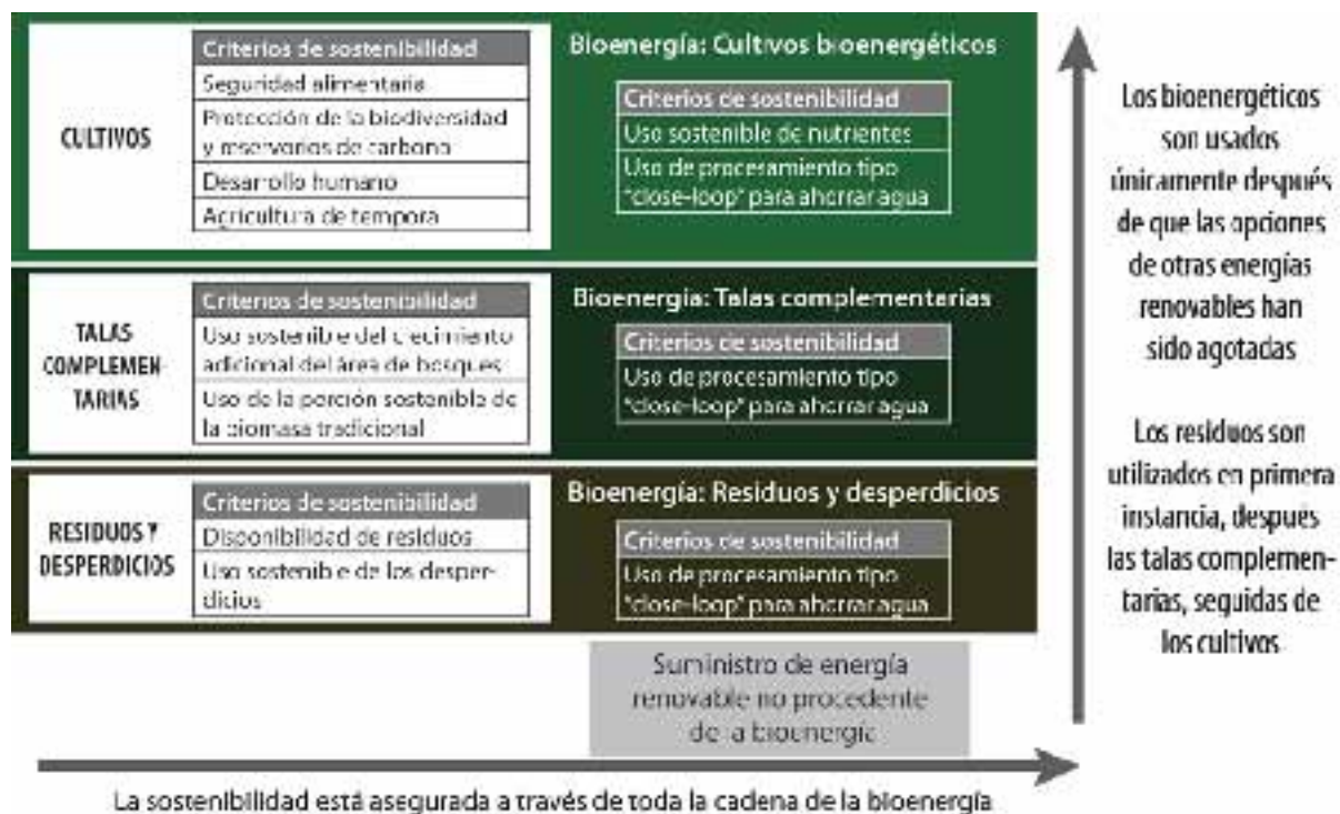
Gráfica 2 – 5 Esquema aplicado en el Escenario Energético para asegurar la sostenibilidad en la oferta de bioenergéticos. (NEl tamaño de las formas en la imagen no es indicativo de la importancia de las categorías en el Escenario)
