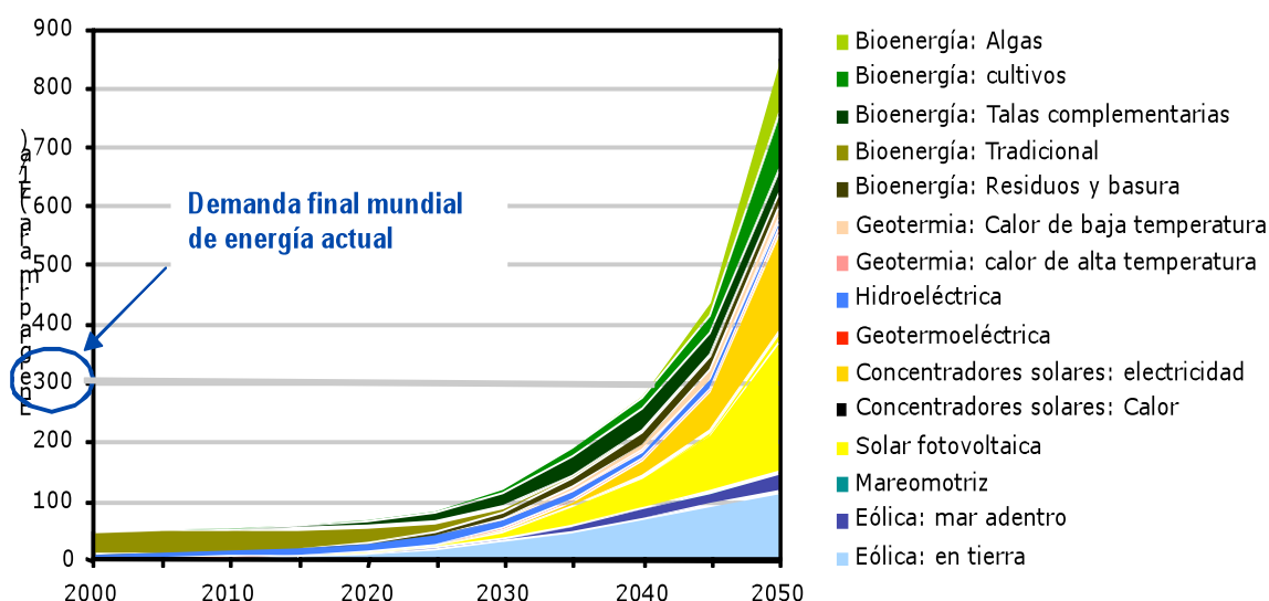
Gráfica 1 – 1 Uso potencial global de varias fuentes de energía renovable.
