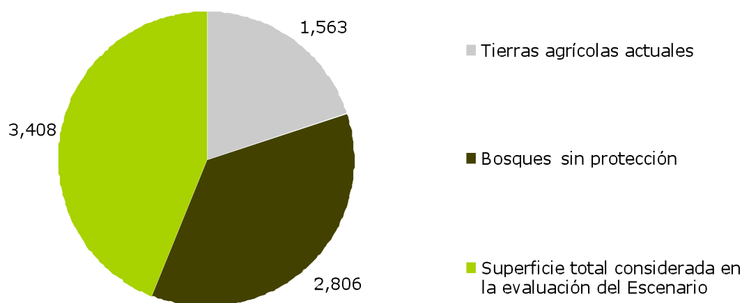
Gráfica 5 – 8 Exclusiones de usos de suelo del Escenario con base en el uso agrícola y las áreas sin protección actuales.
