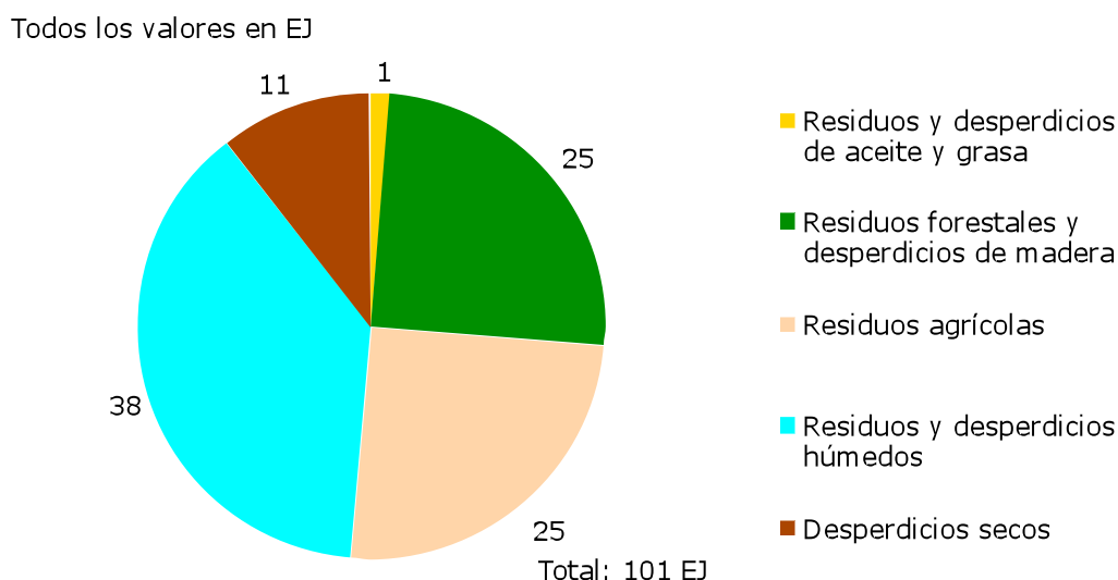
Gráfica 5 – 15 Potencial de residuos y desperdicios sostenibles encontrados en el Escenario a 2050, en cinco categorías. 54
