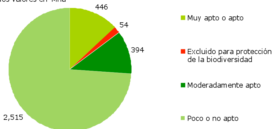
Gráfica 5 – 10 Exclusiones de uso de suelo para el Escenario con base en la protección de la biodiversidad.
