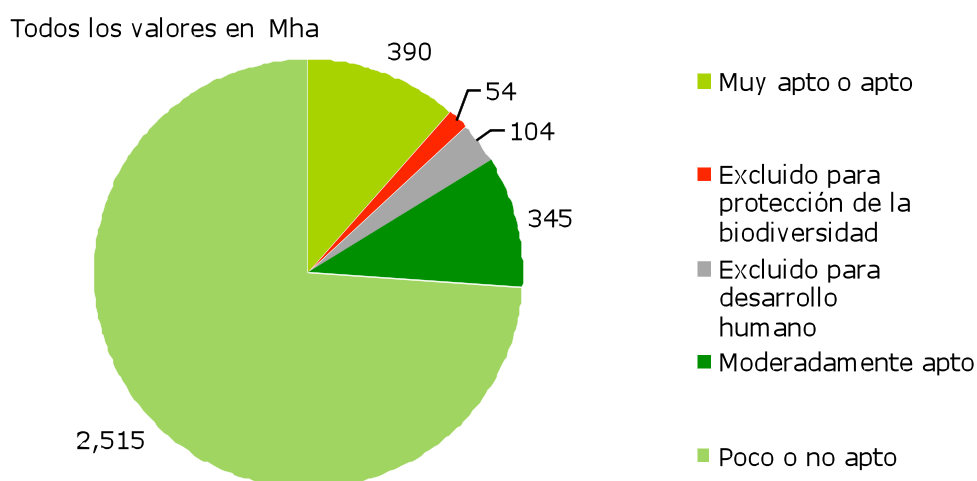
Gráfica 5 – 11 Exclusiones de uso de suelo en el Escenario con base en el desarrollo humano.
