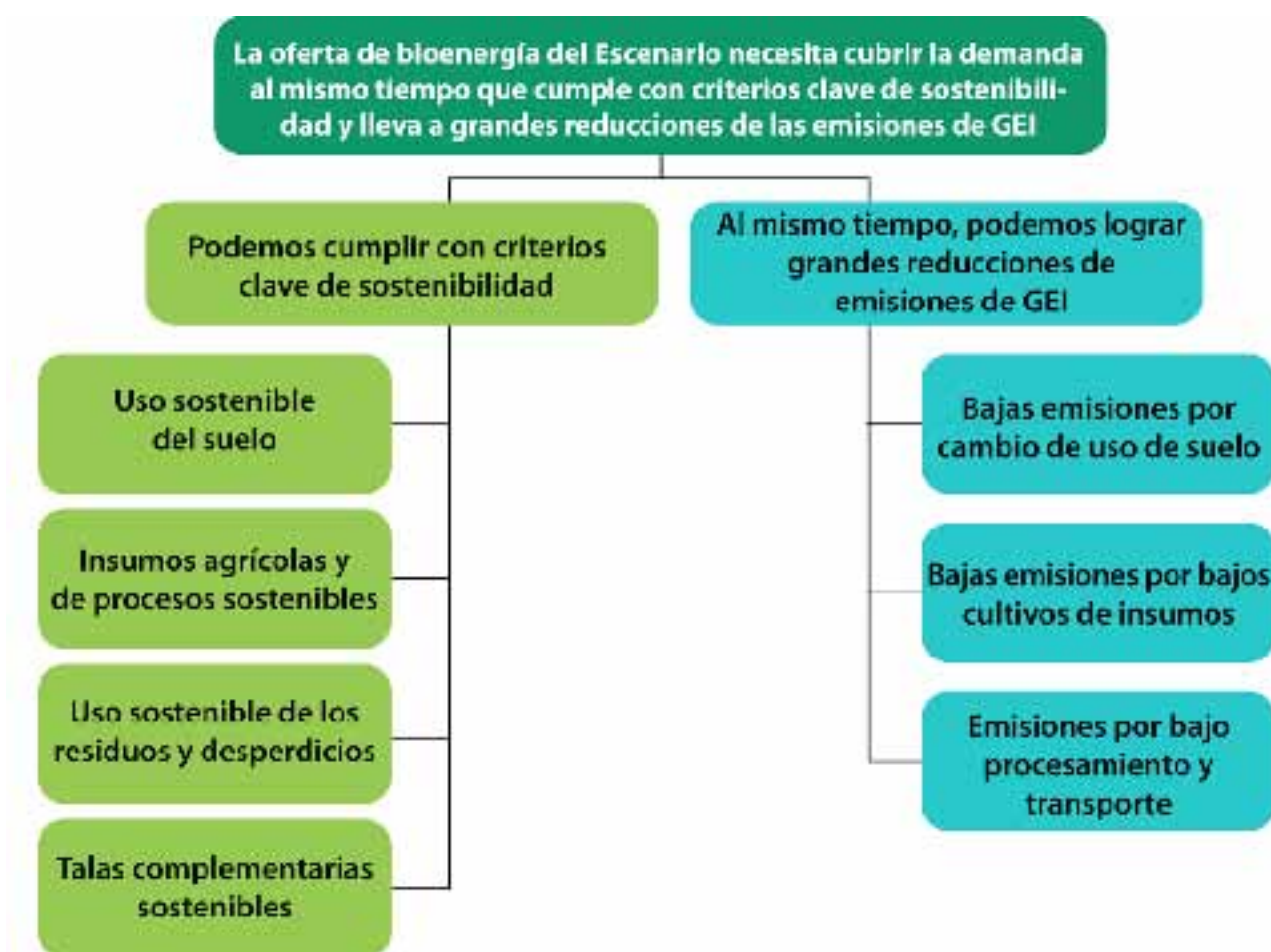
Gráfica 5 – 4 Enfoque conceptual utilizado en el Escenario Energético respecto de la sostenibilidad de la bioenergía.
