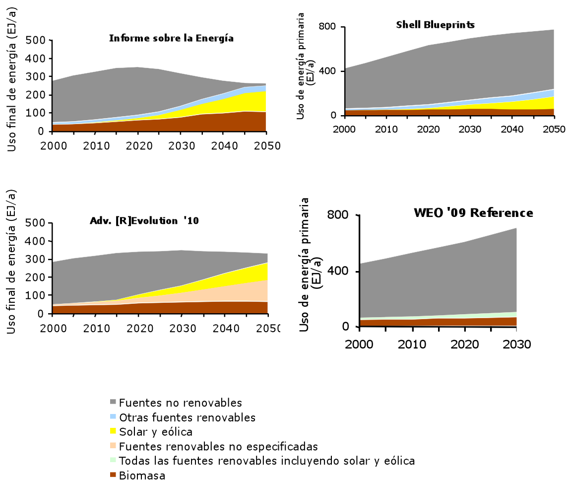
Gráfica 5 – 2 Panorama de la participación de las energías renovables en el Escenario Energético y otros estudios. Los números absolutos no pueden ser comparados entre las dos gráficas de la izquierda y las dos de la derecha, dado que expresan uso de energía final y uso de energía primaria, respectivamente.
