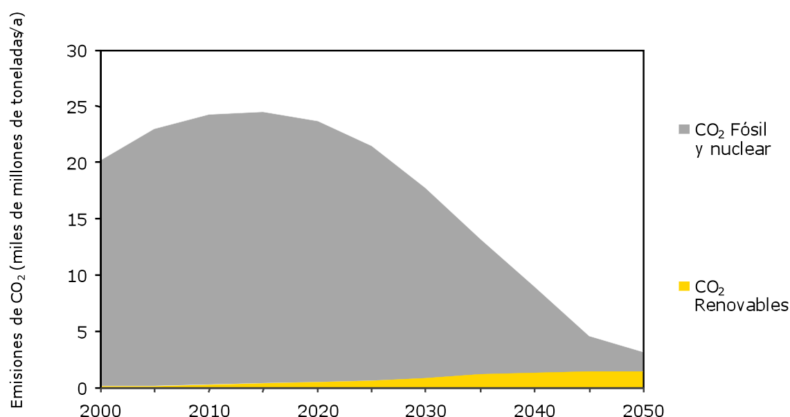
Gráfica 4 – 14 Emisiones globales de CO 2 equivalente como resultado del sistema energético expuesto en el Escenario.
