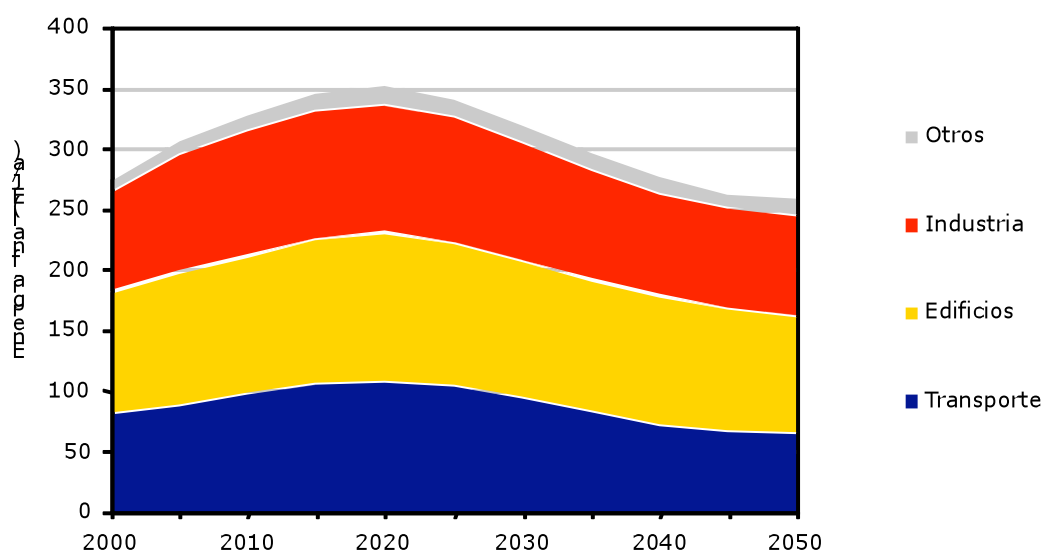
Gráfica 3 – 1 Demanda global de energía en todos los sectores, 2000 a 2050.
