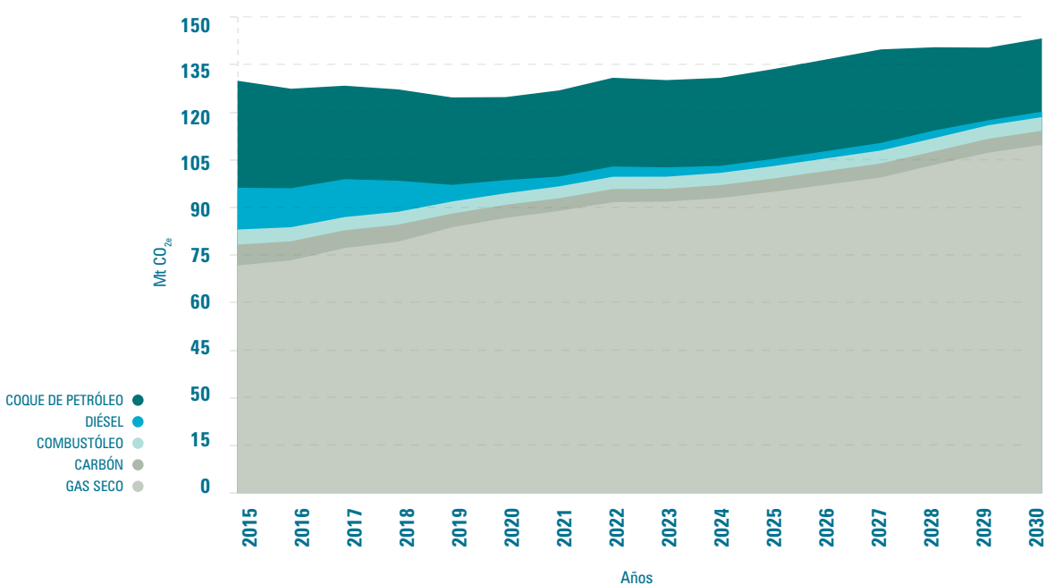
FIGURA 6. EMISIONES DE GEI CORRESPONDIENTES A LA EXPANSIÓN DEL SEN EN PRODESEN 2016-2030 (ORDEN DE MÉRITO)
