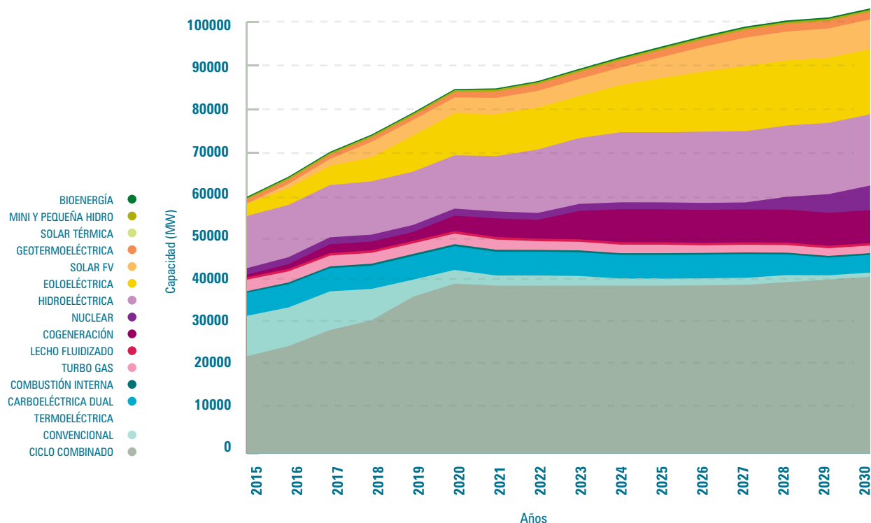
FIGURA 10. EXPANSIÓN DE LA CAPACIDAD INSTALADA EN PRODESEN 2016-2030
