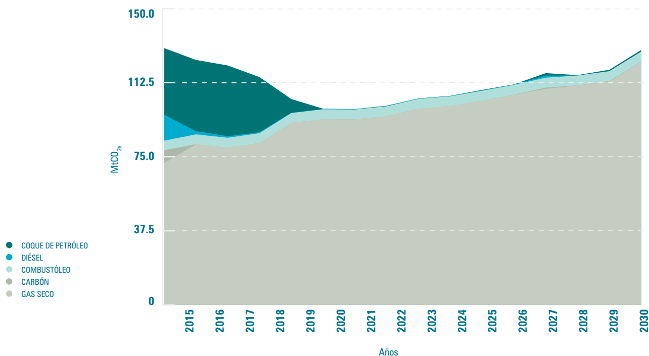
FIGURA 4. EMISIONES DE GEI CORRESPONDIENTES A LA EXPANSIÓN DEL SEN EN PRODESEN 2016-2030 (OPTIMIZADO)
