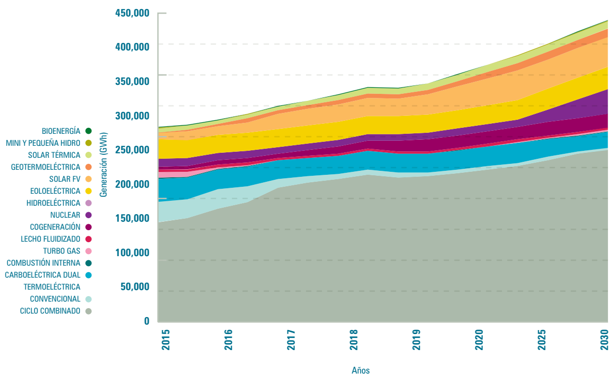
FIGURA 7. GENERACIÓN DE ELECTRICIDAD A PARTIR DE ENERGÍA LIMPIA EN PRODESEN 2016-2030 (ORDEN DE MÉRITO)
