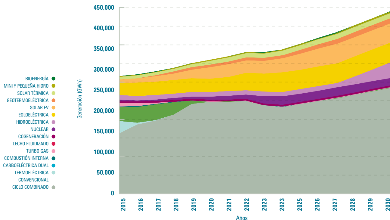
FIGURA 5. GENERACIÓN DE ELECTRICIDAD A PARTIR DE ENERGÍA LIMPIA EN PRODESEN 2016-2030 (OPTIMIZADO)
