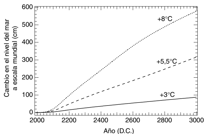
Figura 27: Respuesta de la capa de hielo de Groenlandia en tres escenarios de calentamiento climático durante el tercer milenio, expresada en cambios equivalentes en el nivel del mar a escala mundial. Los valores asignados a las curvas corresponden al aumento de la temperatura media anual en Groenlandia para el año 3000 D.C., de acuerdo con las predicciones de un modelo climático y oceánico bidimensional forzado con aumentos en la concentración de GEI hasta el año 2130 D.C., la que se mantiene constante después de esa fecha. Véase que las temperaturas proyectadas para Groenlandia son en general de 1,2 a 3,1 veces superiores al promedio de las temperaturas a nivel mundial, de acuerdo con los diversos modelos utilizados en el Capítulo 11. [Basado en la Figura 11.16]
