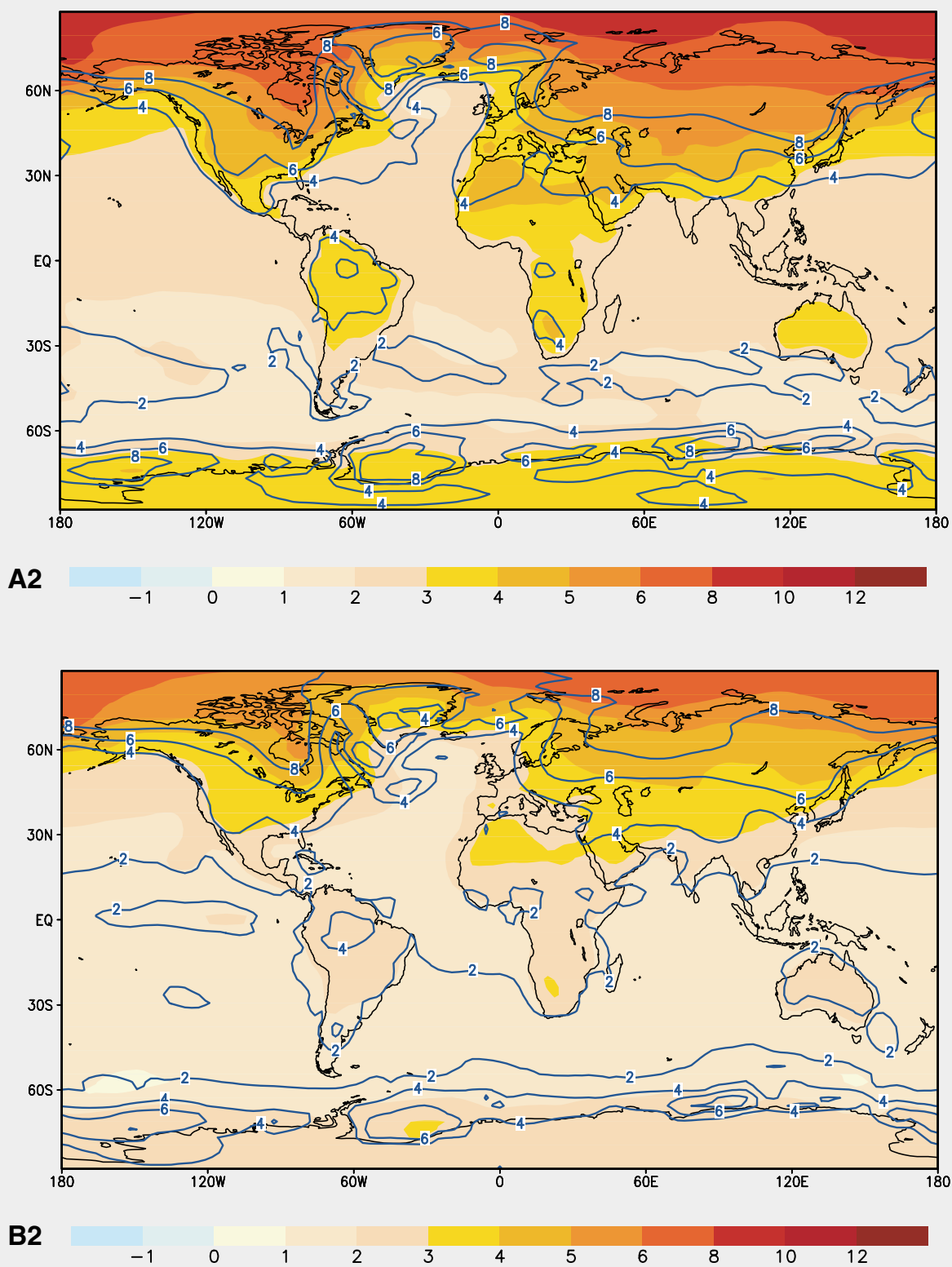
Figura 20: Cambio anual medio de la temperatura (sombreado en colores) y su margen de variación (isolíneas) (Unidad: °C) en el escenario A2 del IE-EE (recuadro superior) y en el escenario B2 del IE-EE (recuadro inferior). Ambos escenarios comparan el período 2071-2100 con el período 1961-1990 y se simularon con MCGAO. [Basado en las Figuras 9.10d y 9.10e]
