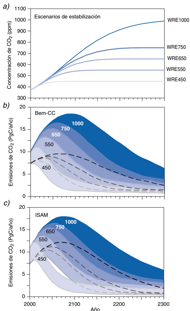
Figura 25: Emisiones de CO 2 proyectadas que permiten estabilizar las concentraciones atmosféricas de CO 2 en distintos valores finales.
